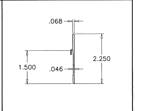
E20 SILL RISER
