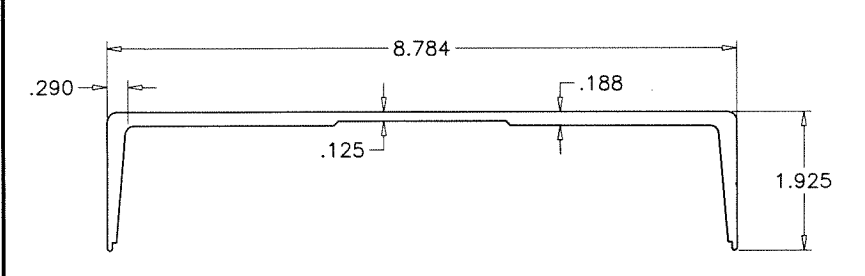
E18 RECEPTOR STIFFENER
