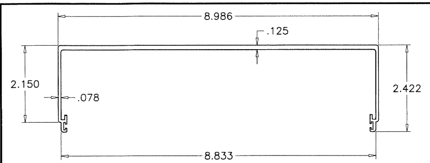
E17 HEAD RECEPTOR
